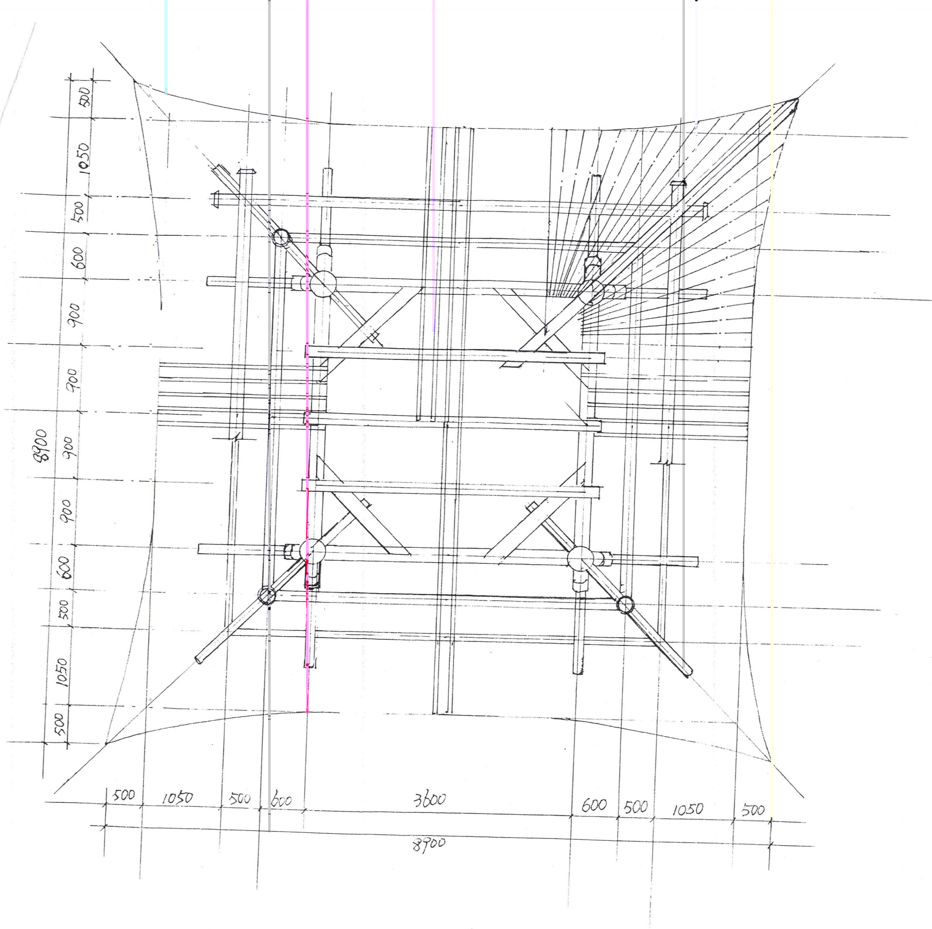
三层结构平面布置图 1:50
