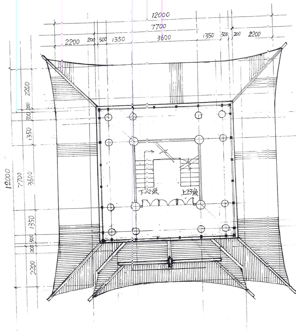
二层平面图 1:100
